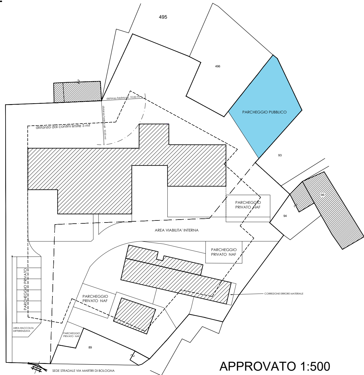
APPROVATO 1:500
